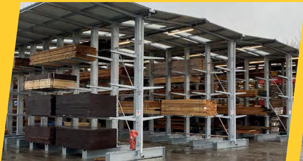
Cantilever : Poids et hauteur selon votre cahier des charges
